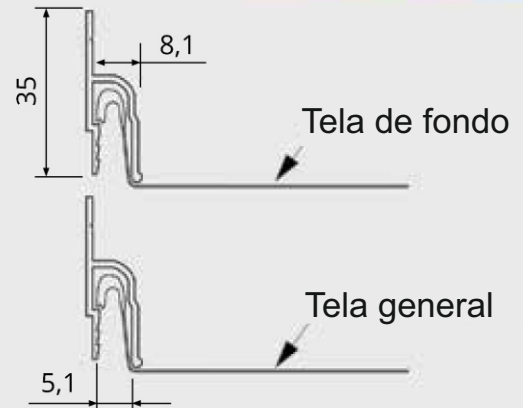
Perfil standard
