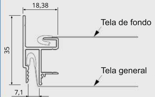
Perfil Apply 20
